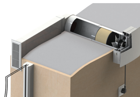
Montaż kątowy z zastosowaniem kanału wentylacyjnego i kolanka 90°
